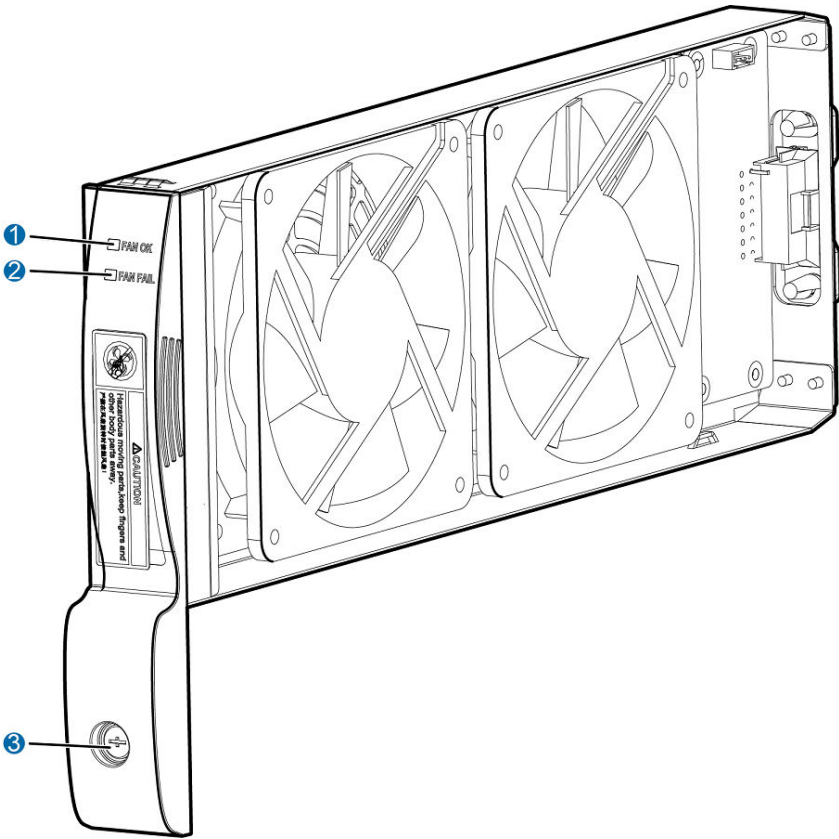
图 3-3 VP9650 风扇框
