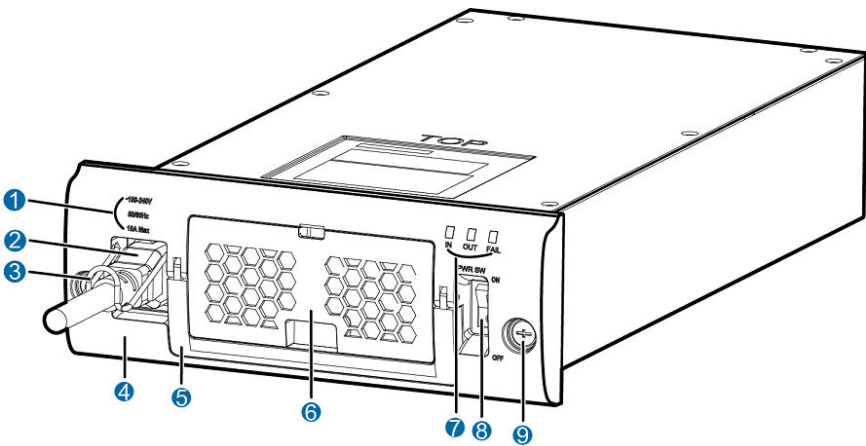
图 3-4 交流电源模块外观模块
