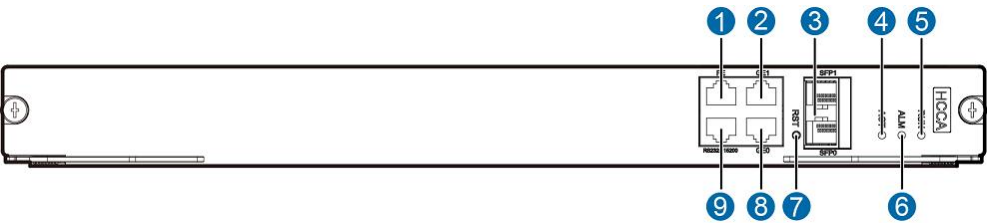
图 3-9 HCCA 单板前面板
