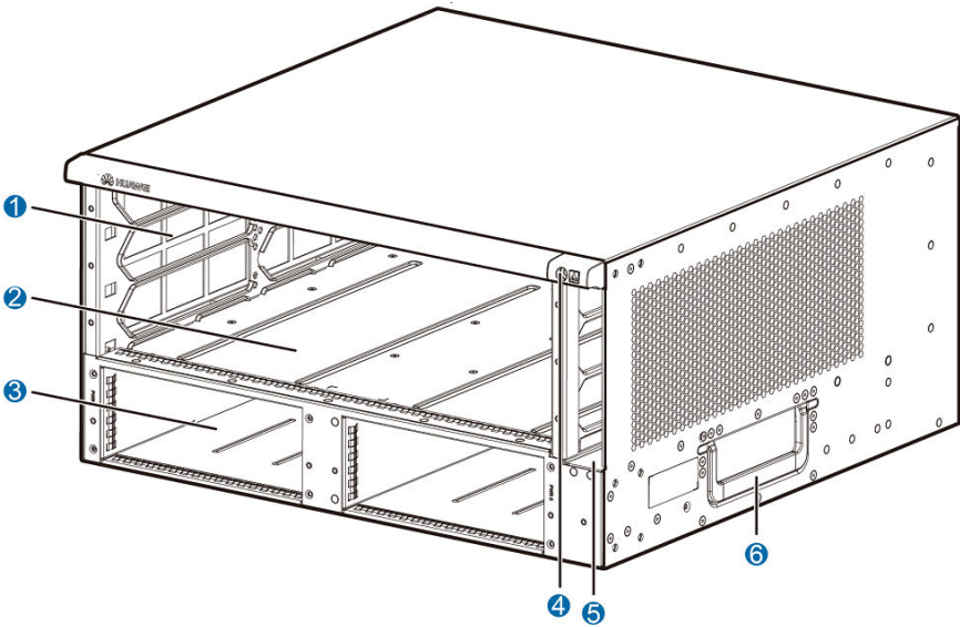
图 3-2 VP9650 机箱整体结构
