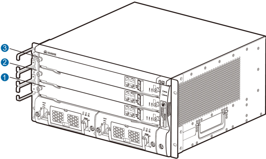
图 3-7 VP9650 单板槽位分布
