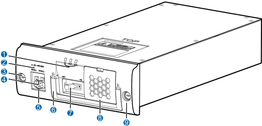
图 3-5 直流电源模块外观模块
